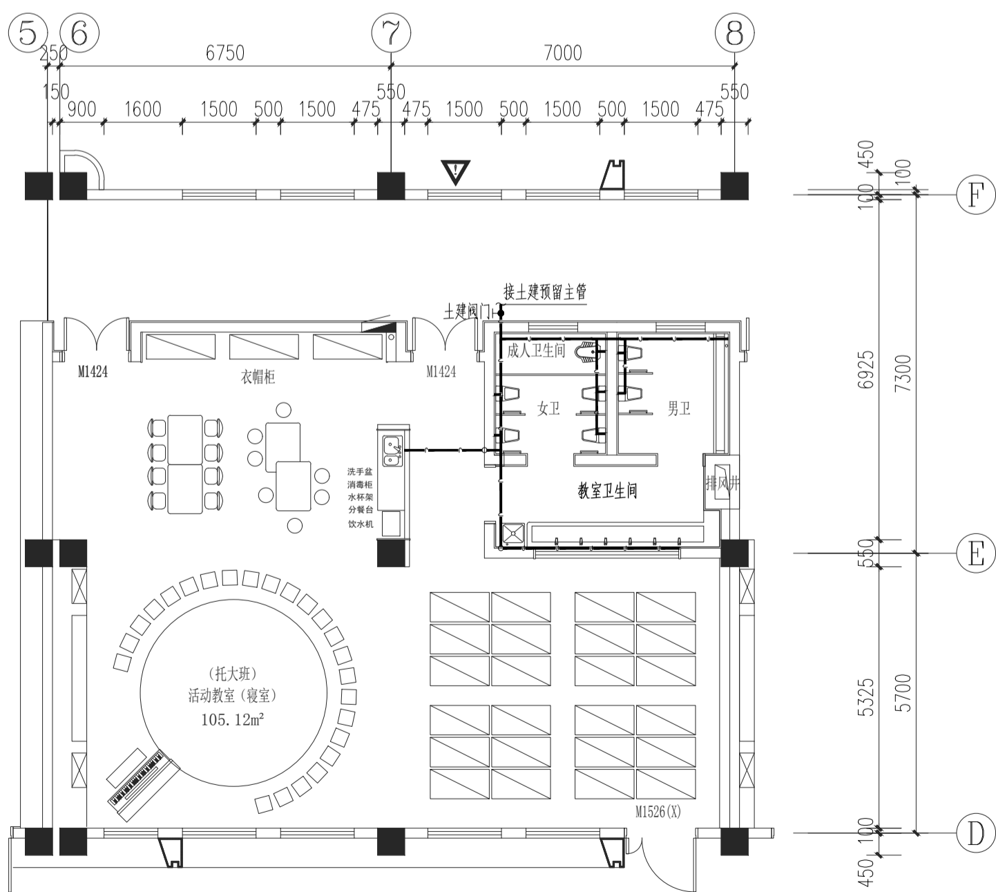
2-3层教室卫生间大样图 1:100
