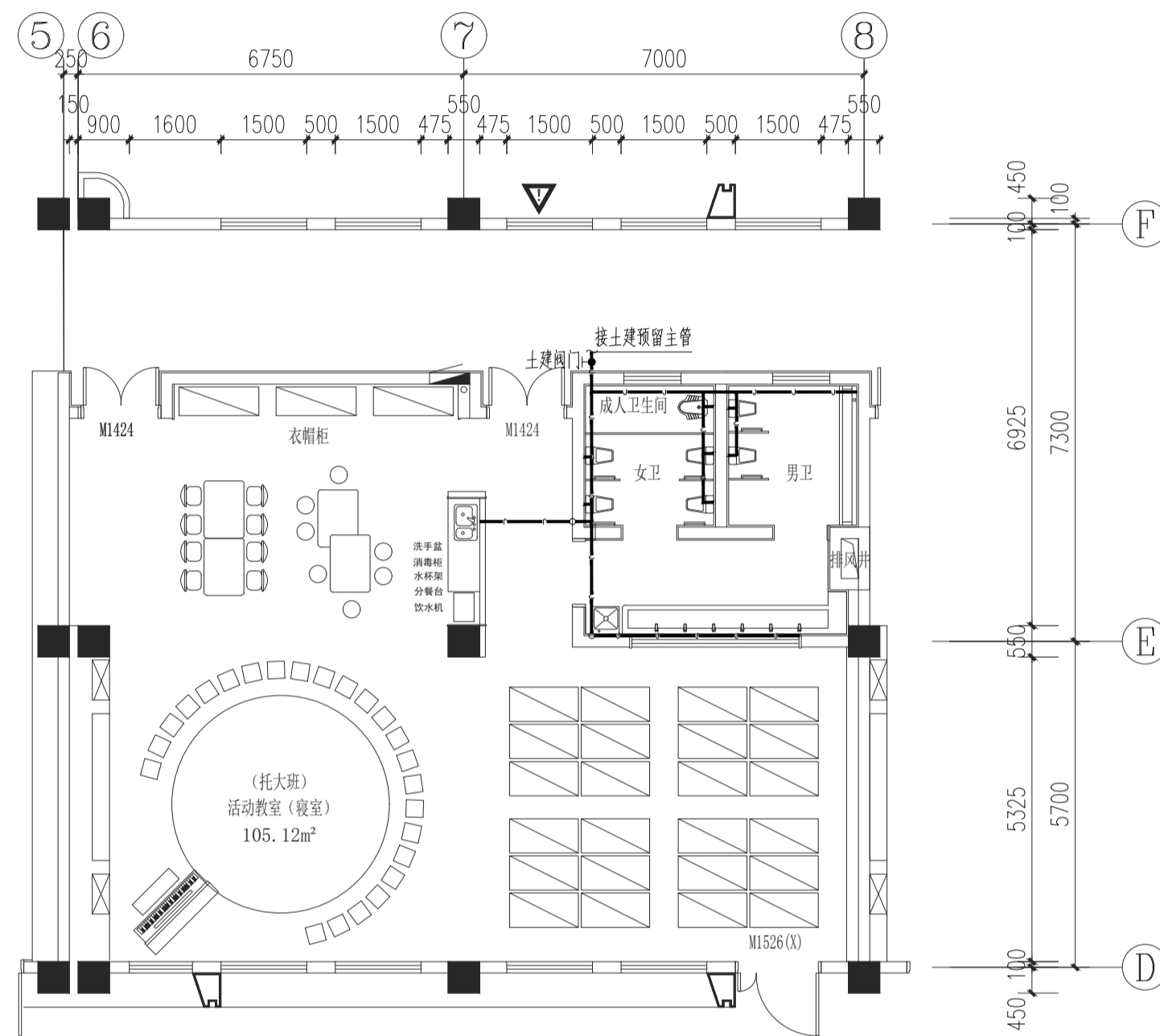
1层教室卫生间大样图 1:100
