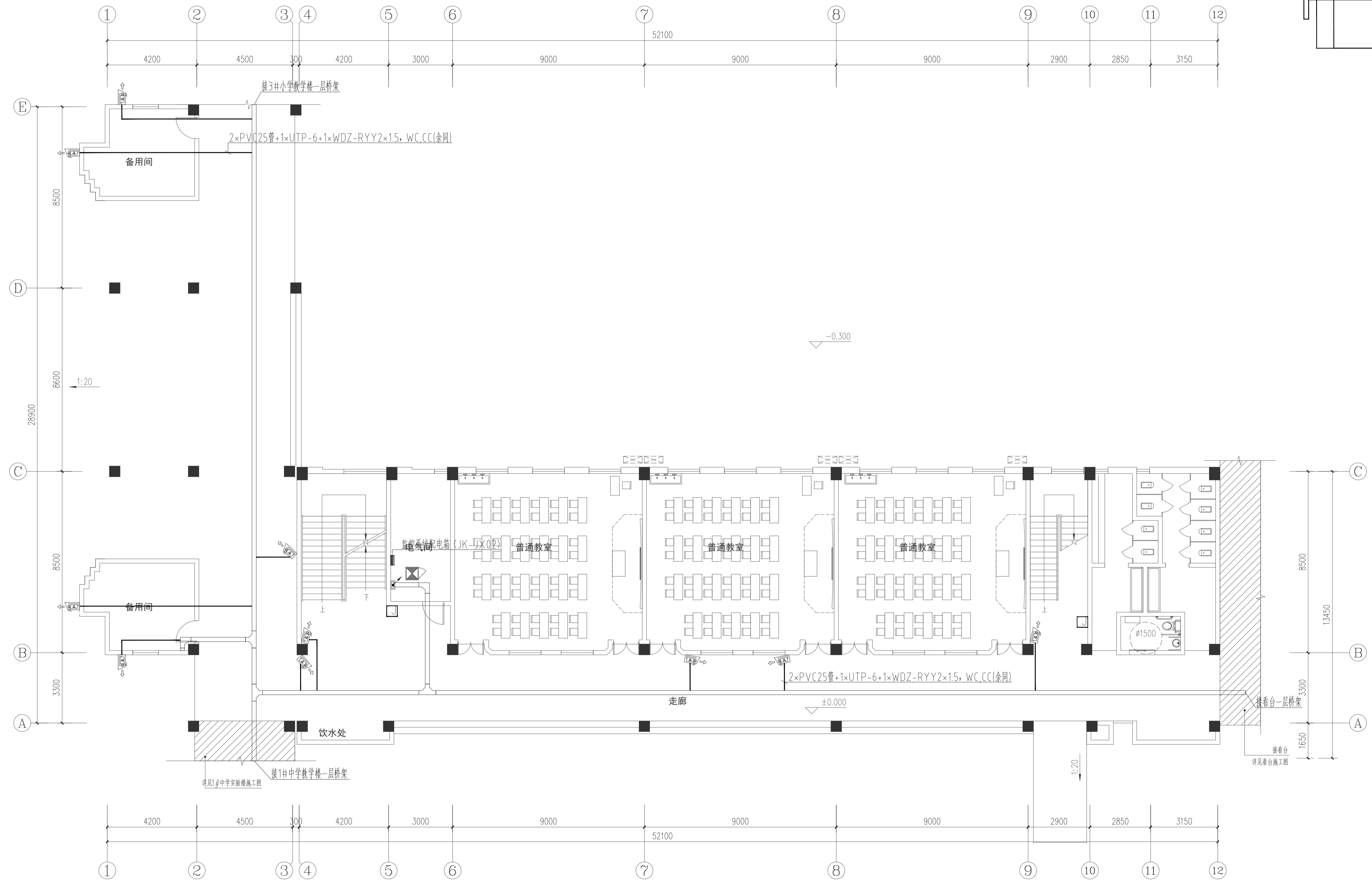
2#中学教学楼一层安防平面图 1:100
