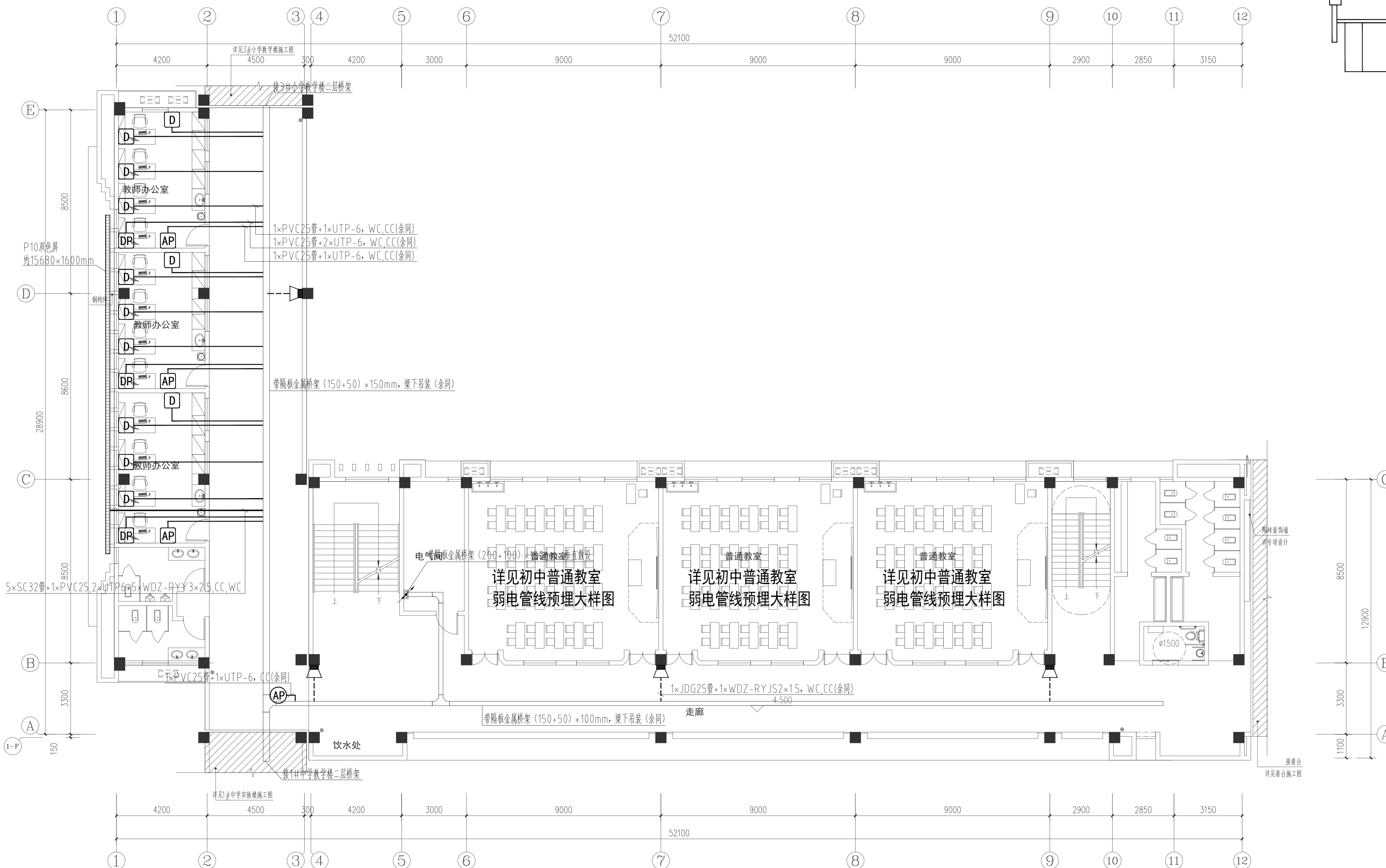
2#中学教学楼二层综合布线平面图 1:100
