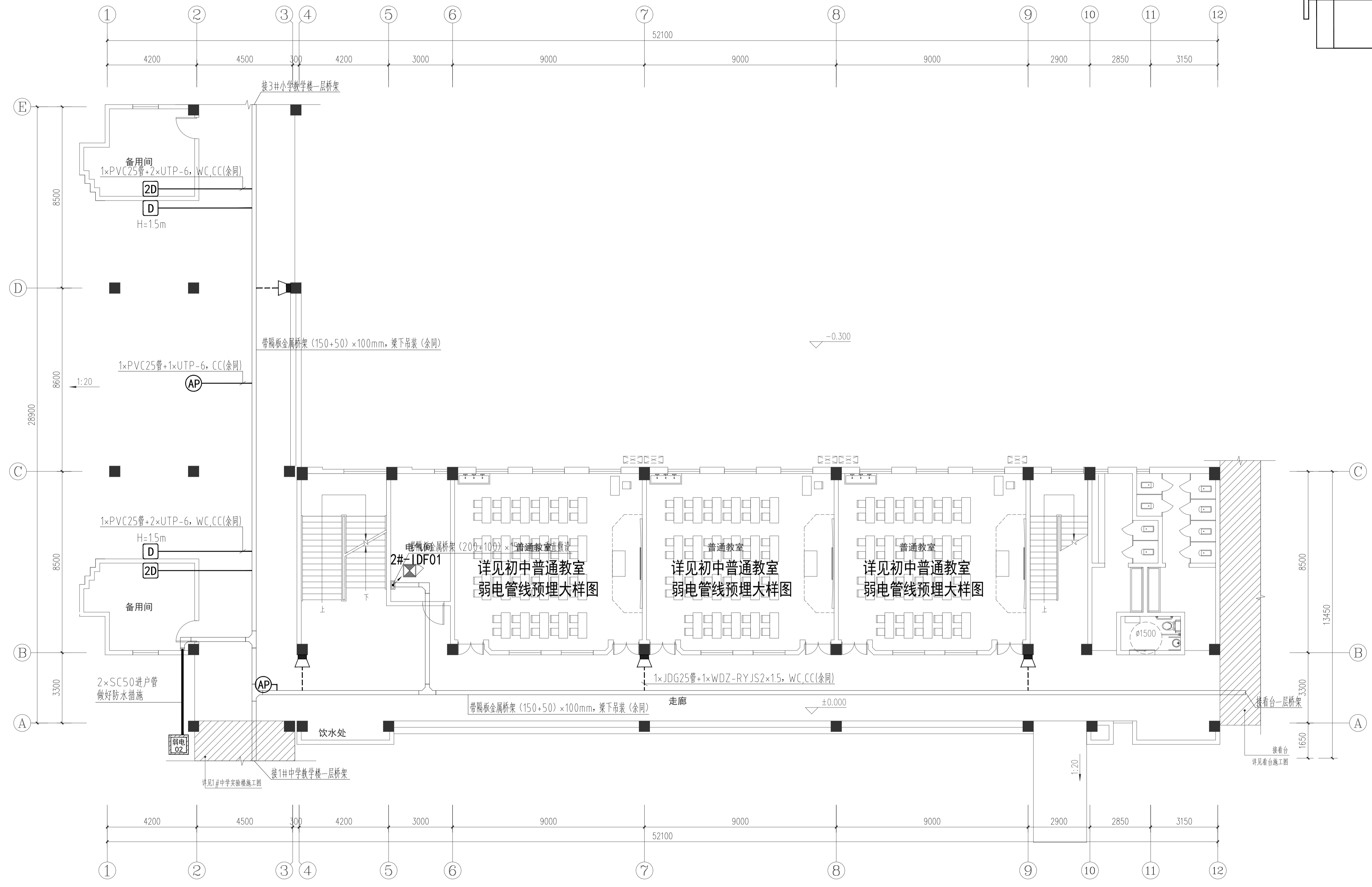
2#中学教学楼一层综合布线平面图 1:100
