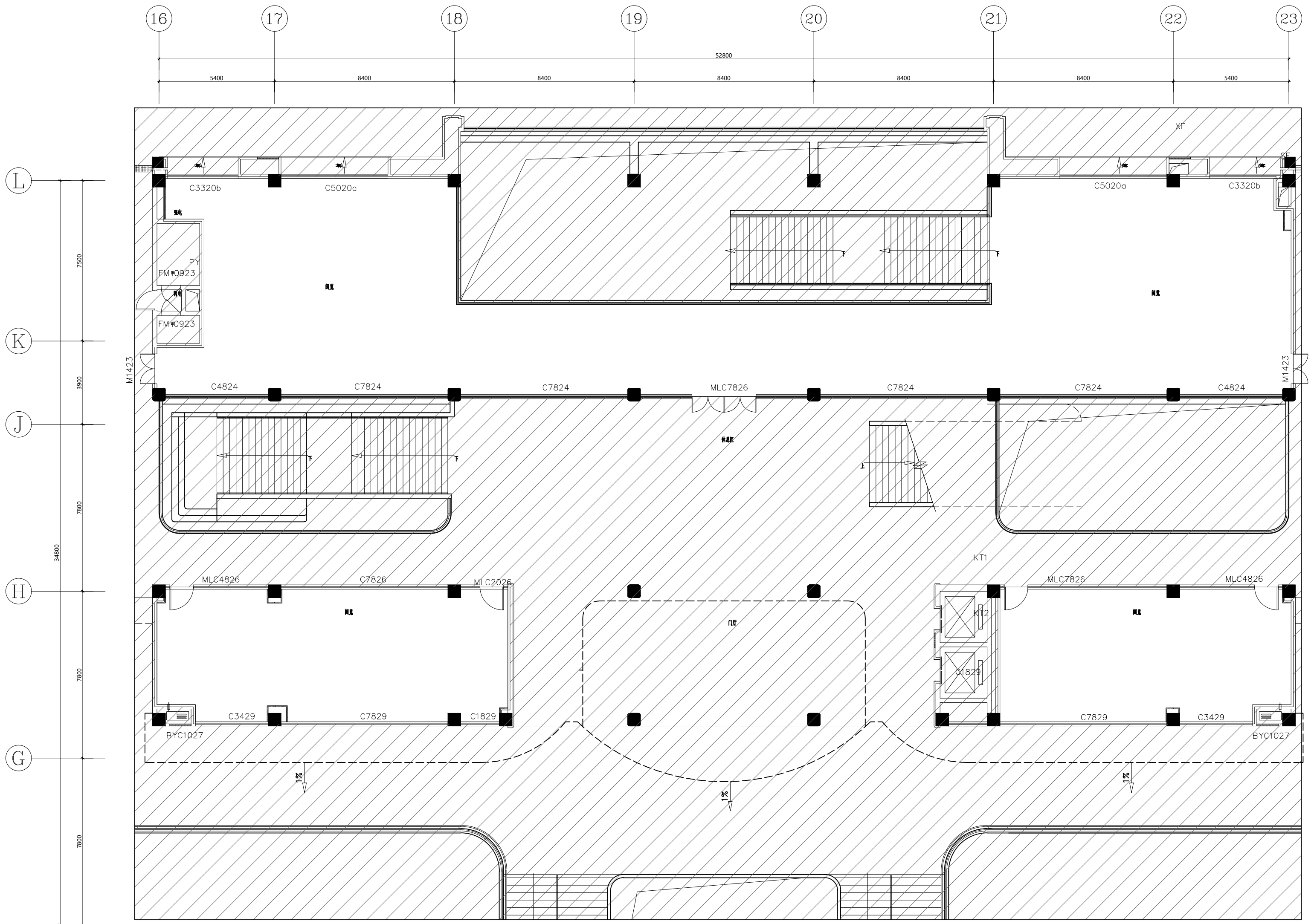
二层原始建筑图
